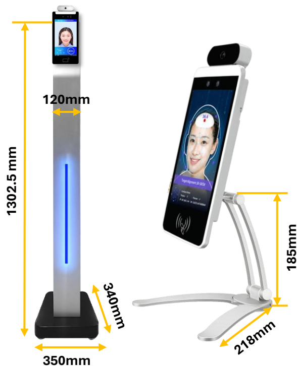
【床設置／卓上スタンドセット】
