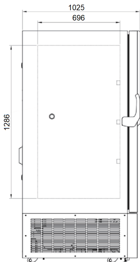
側面図
